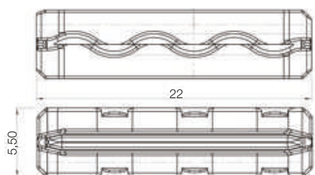
MARC adaptador para montaje lateral en contactores WEG
