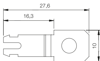
Adaptador PLMP
