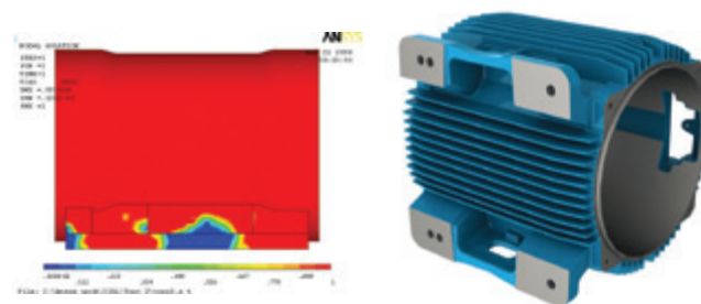
Figura 5 - Patas sólidas
