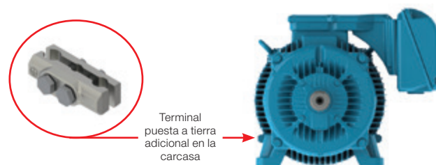
Figura 9 - Disposición de los terminal puesta a tierra adicional en la carcasa.
