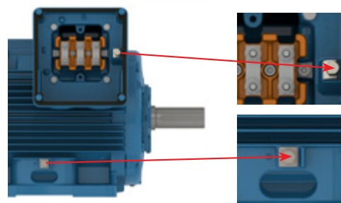
Figura 8 - Terminales de puesta a tierra en la caja de conexiones y en la carcasa
