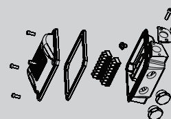
Kit de Caja de Conexión Auxiliar
