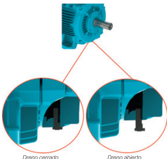
Figura 17 - Detalle del drenaje en la tapa delantera
