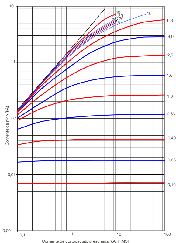
Curva de Limitación de Corriente en Cortocircuito en 500 V - MPW40
